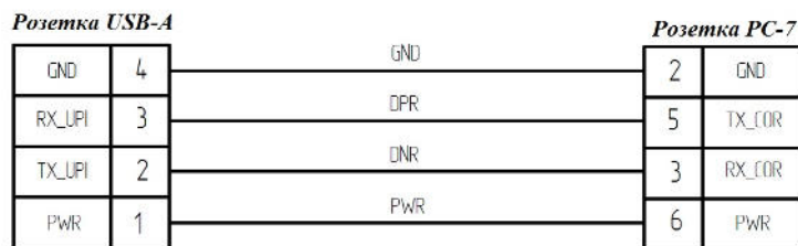
Рисунок 2 – Схема розпайки кабелю
