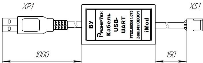
Рисунок 2 – Кабель для підключення до комплексу вимірювального КВУ: модифікація USB–UART– РС
