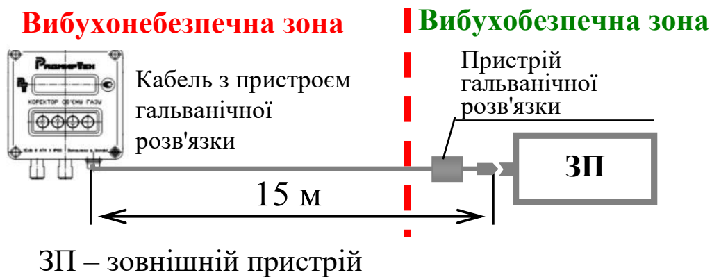
Рисунок 1 - Схема підключення кабелю з пристроєм гальванічної розв'язки
