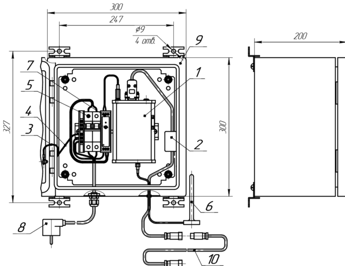
Рисунок 2 - Зовнішній вигляд, габаритні та приєднувальні розміри модуля
