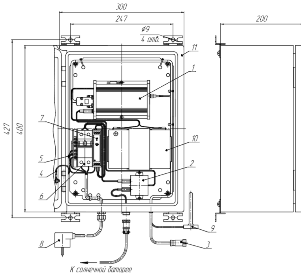
Рисунок 3 - Зовнішній вигляд, габаритні та приєднувальні розміри модуля
