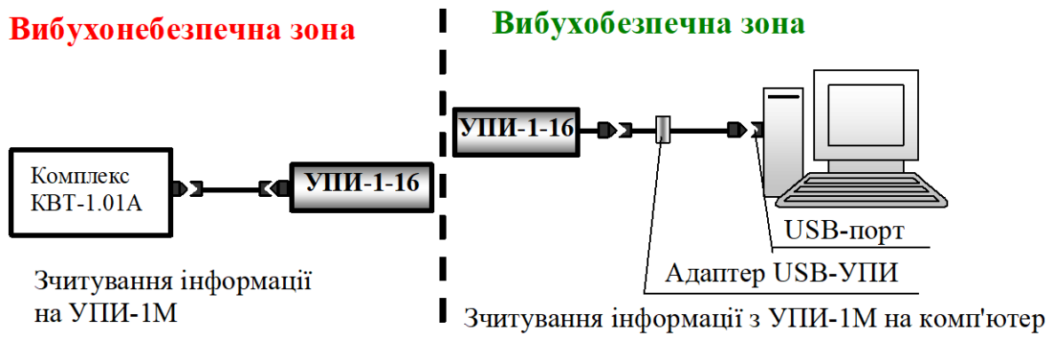
Рисунок 12.11 – Зчитування інформації з Комплексу КВТ-1.01А виконання 00 за допомогою УПИ-1-16
