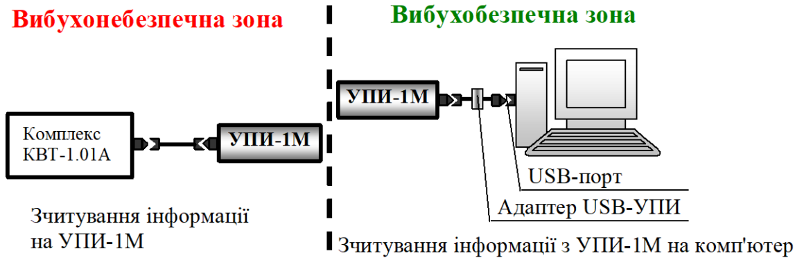
Рисунок 12.10 – Зчитування інформації з Комплексу КВТ-1.01А модифікації 00 за допомогою УПИ-1М
