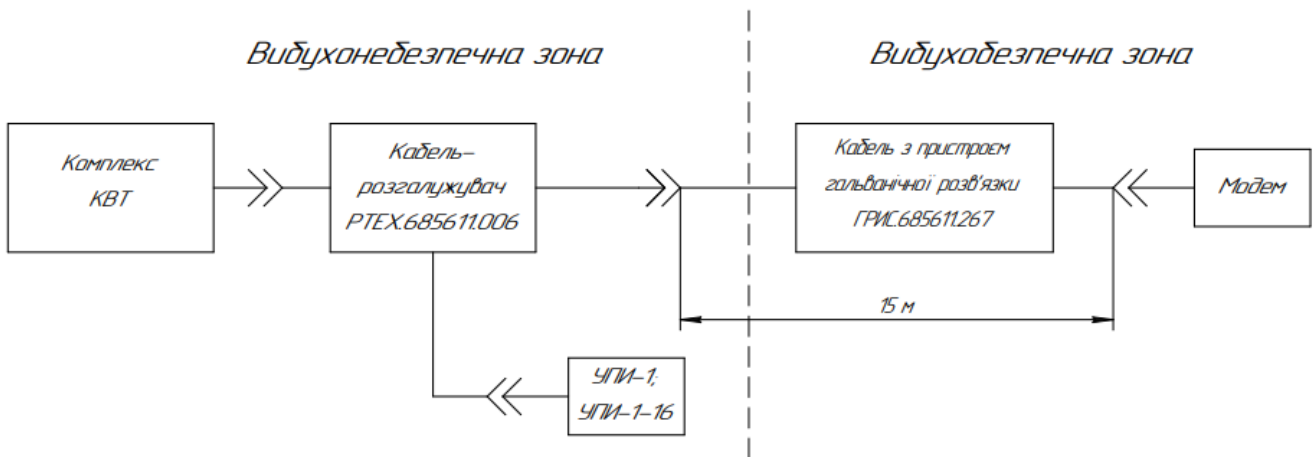
Рисунок 12.12 – Підключення УПІ-1М та УПІ-1-16 до Комплексу КВТ–1.01А виконання 00 за допомогою кабелю розгалужувача.
