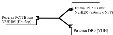
Рисунок 1 – Схема кабеля– розгалужувача КР-006
