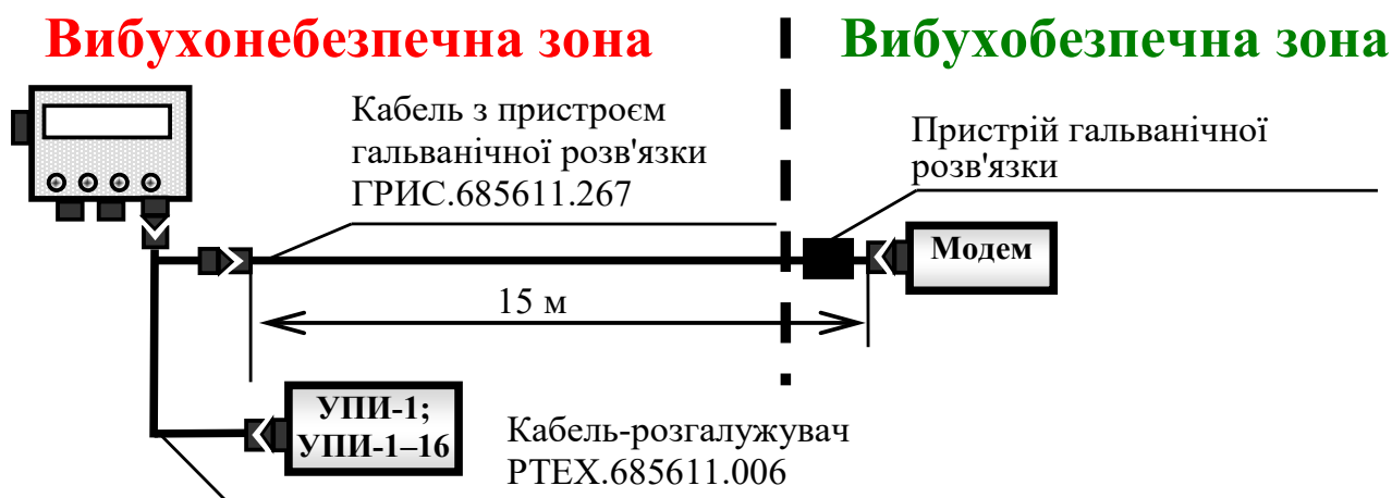
Рисунок 2 – Схема підключення кабелю-розгалужувача КР–006
