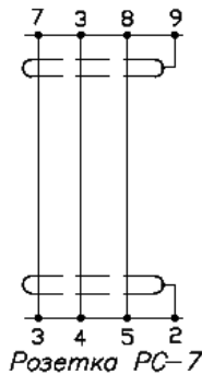
Рисунок 2 – Схема розпайки кабелю до УПИ
