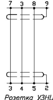
Рисунок 2 – Схема розпайки кабелю до УПИ
