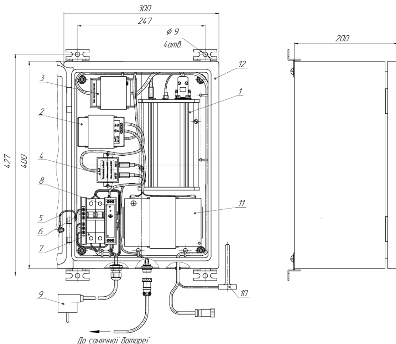
Рисунок 3 - Зовнішній вигляд, габаритні та приєднувальні розміри модуля
