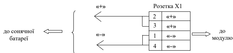
Рисунок 4 - Схема розпайки кабелю підключення сонячної батареї к модулю
