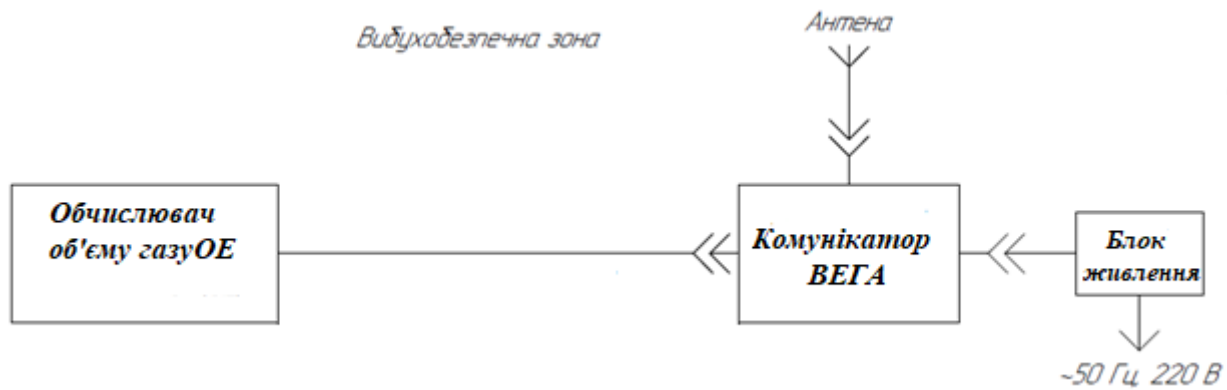
Рисунок 3 – Схема підключення комунікатора ВЕГА до обчислювача об'ємної витрати і об'єму газу ОЕ-22ЛА
