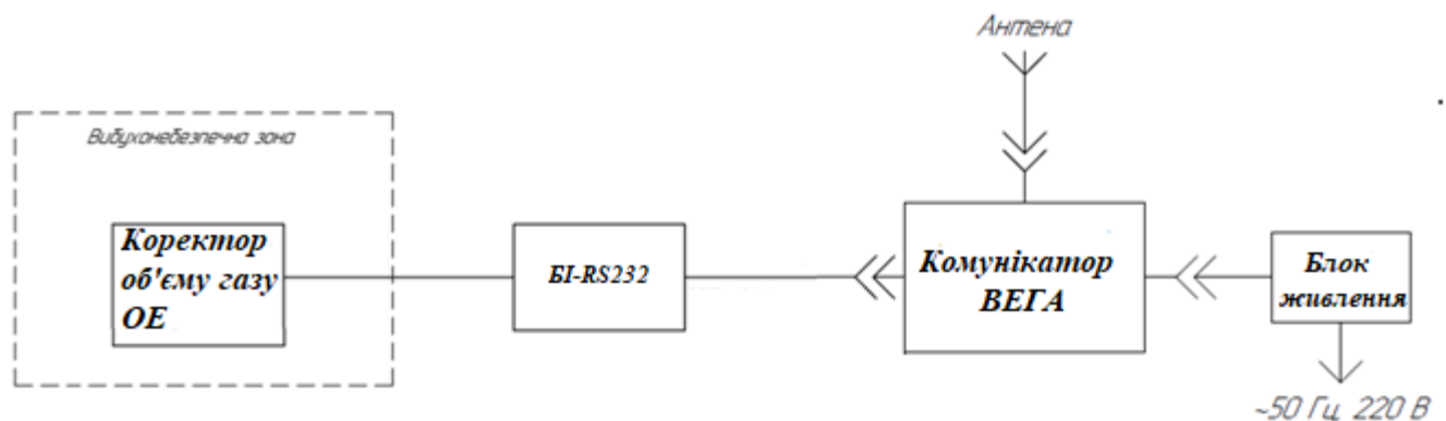
Рисунок 2 – Схема підключення комунікатора ВЕГА до коректора об'єму газу ОЕ
