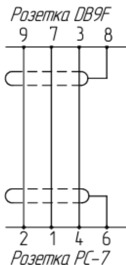
Рисунок 2 – Схема розпайки кабелю до УПИ
