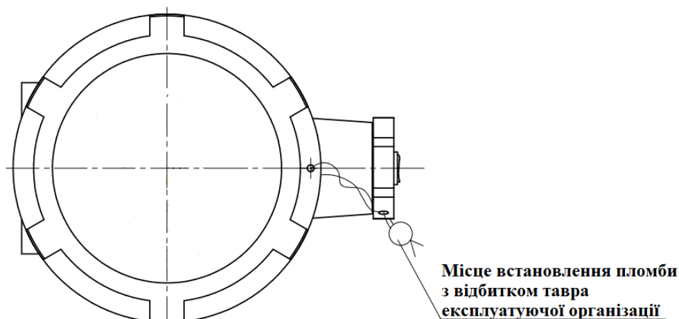
Рисунок 9 – Схема пломбування кришки перетворювача
