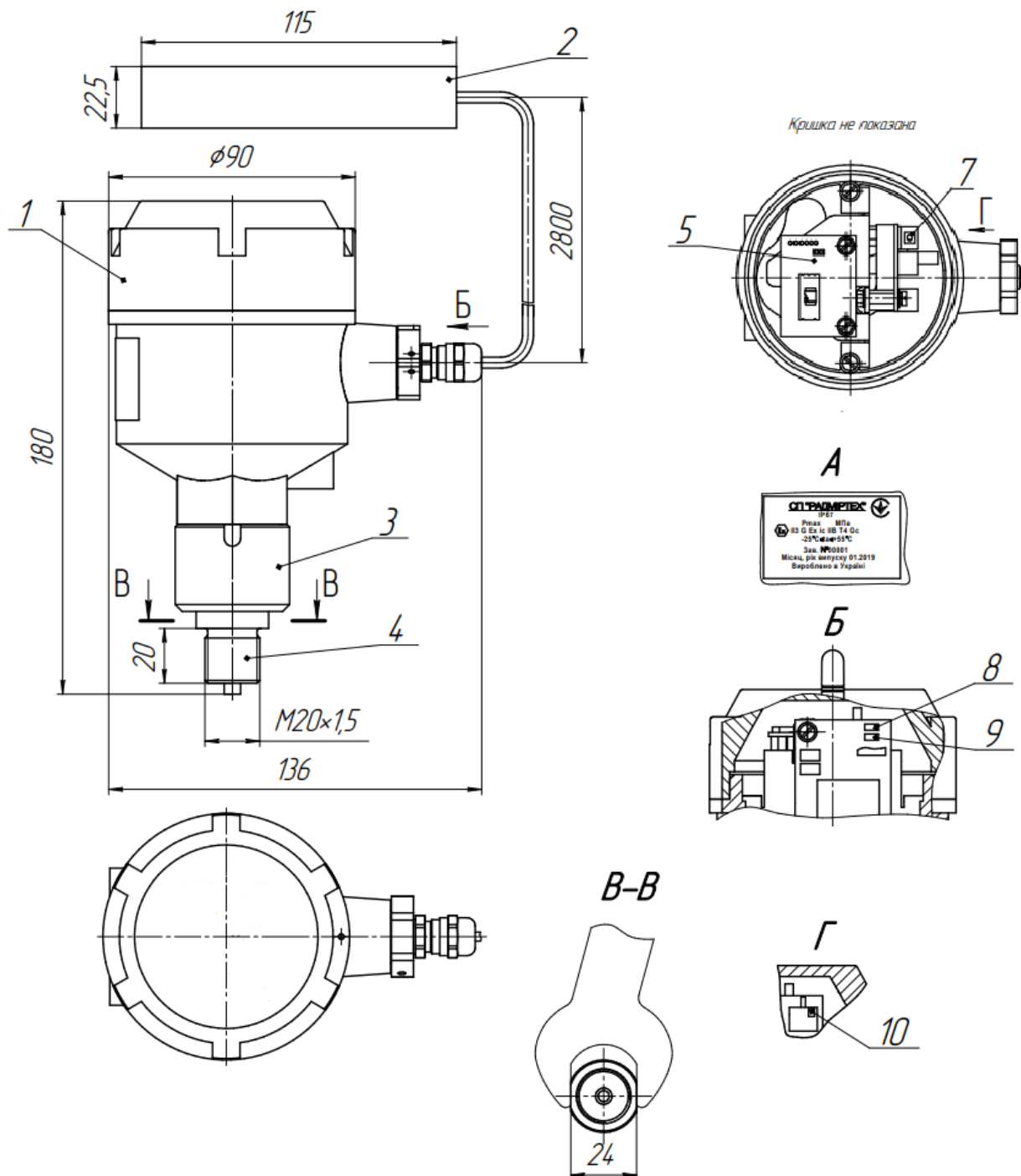
Рисунок 3 – Зовнішній вигляд, габаритні та приєднувальні розміри перетворювача надлишкового тиску з вбудованим GSM-модемом ВЕГА-ДИ-GSM-1
