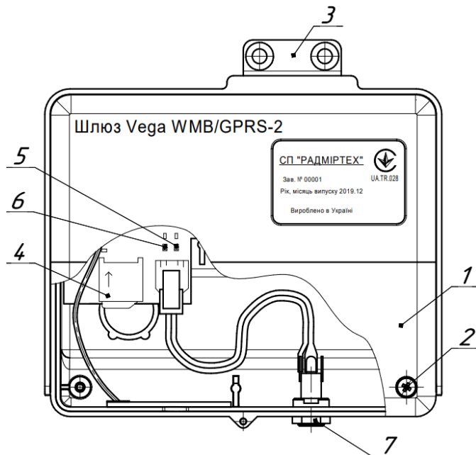
Рисунок 5 - Зовнішній вигляд шлюза Vega WMB/GPRS-2
