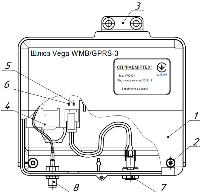
Рисунок 6 - Зовнішній вигляд шлюза Vega WMB/GPRS-3
