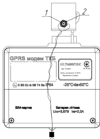
Рисунок 4 – Місце пломбування GPRS модему ТКБ-CAMГАЗ, ТКБ-Pietro Fiorentini
