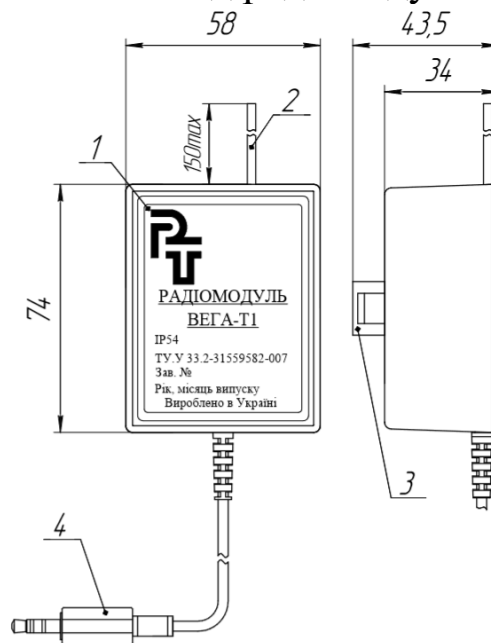
Рисунок А.1 – Зовнішній вигляд радіомодулю ВЕГА-Т ретранслятор
