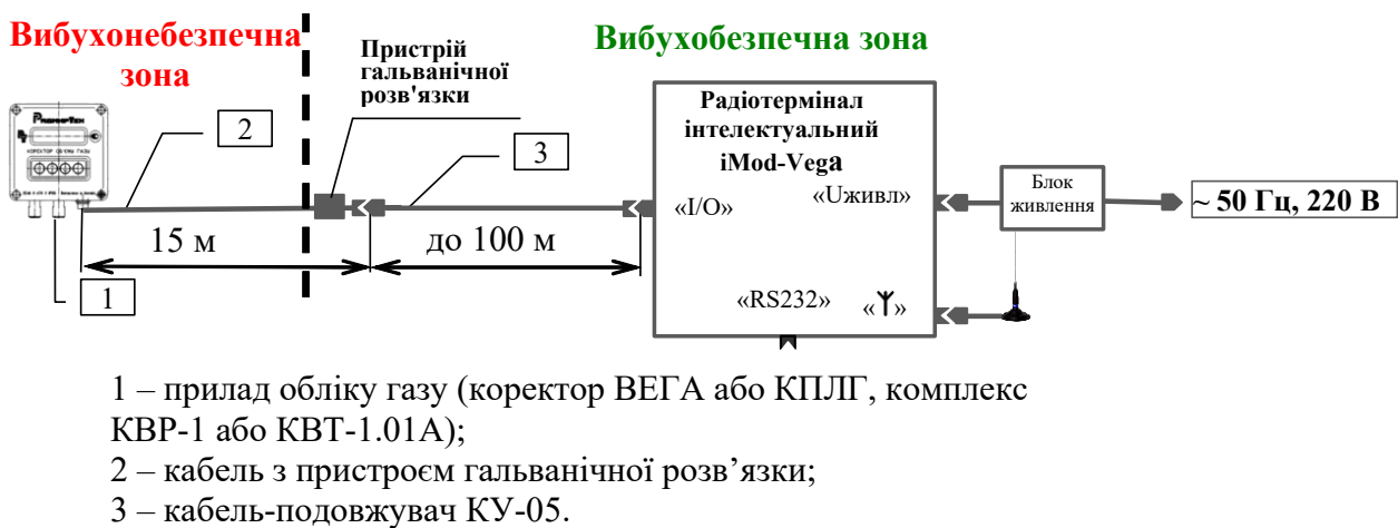
Рисунок 2 – Схема підключення радіотерміналу
