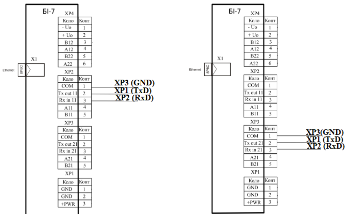
Рисунок 3 – Нумерація контактів з'єднувачей для підключення кабелю РТЕХ.685611.047
