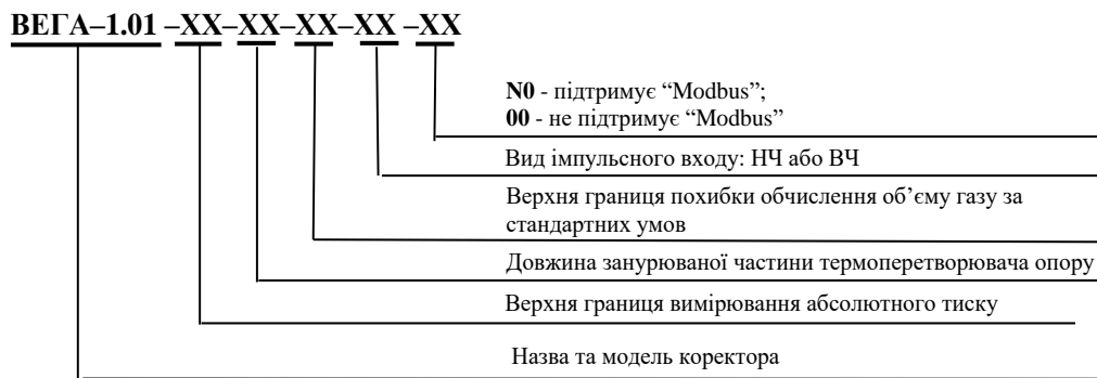
Рисунок 1 – Схема складання умовного позначення коректору БЕГА-1.01
