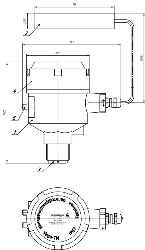
Рисунок 6 – Зовнішній вигляд та габаритні розміри терміналу багатофункціонального Vega-TM-7
