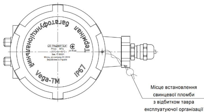
Рисунок 14 – Схема пломбування терміналу багатофункціонального Vega-TM-0, терміналу багатофункціонального Vega-TM-1 та терміналу багатофункціонального Vega-TM-7
