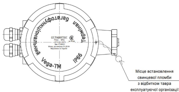
Рисунок 14 – Схема пломбування терміналу багатофункціонального Vega-TM-0, терміналу багатофункціонального Vega-TM-1 та терміналу багатофункціонального Vega-TM-7
