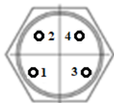
Рисунок 10 – Схема підключення терміналу багатофункціонального Vega-TM-0 та терміналу багатофункціонального Vega-TM-7.
