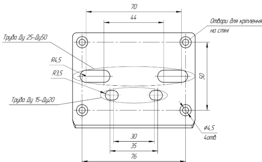
Рисунок 9 – Кронштейн для кріплення терміналу Vega-TM-7
