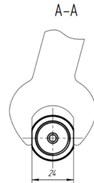
Рисунок 2 – Зовнішній вигляд та габаритні розміри термінала багатофункціонального Vega-TM-0.
