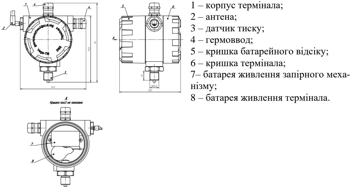
Рисунок 4 – Зовнішній вигляд та габаритні розміри термінала багатофункціонального Vega-TM-2, термінала багатофункціонального Vega-TM-6
