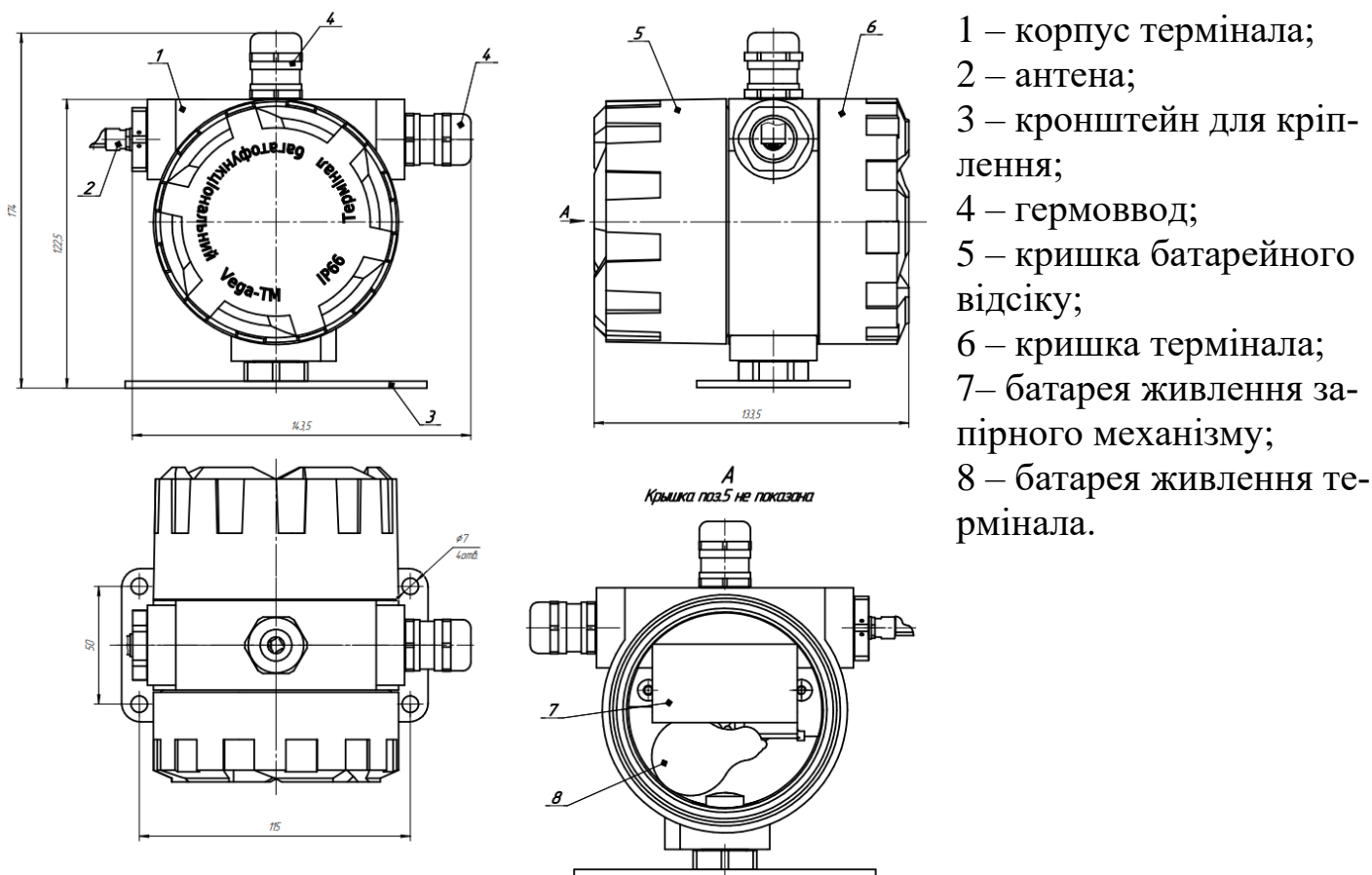
Рисунок 5 – Зовнішній вигляд та габаритні розміри термінала багатофункціонального Vega-TM-3, термінала багатофункціонального Vega-TM-4, термінала багатофункціонального Vega-TM-5
