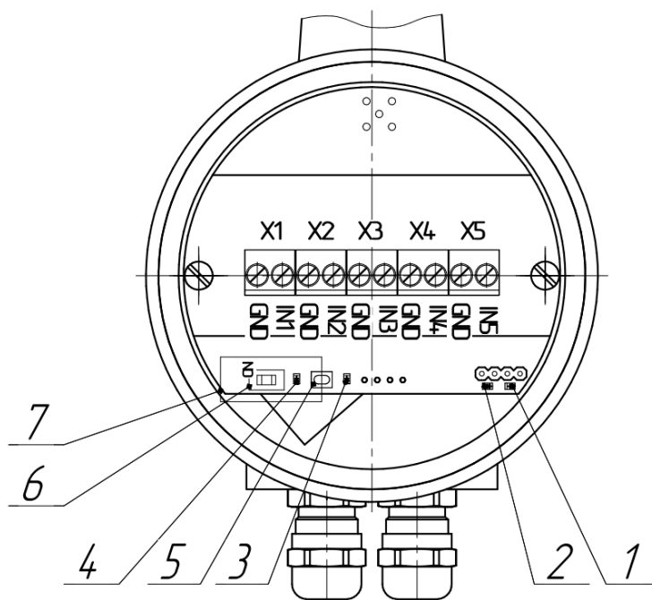
Рисунок 12 – Розміщення клем підключення термінала багатофункціонального Vega-TM-1
