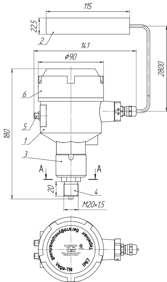
Рисунок 2 – Зовнішній вигляд та габаритні розміри термінала багатофункціонального Vega-TM-0.
