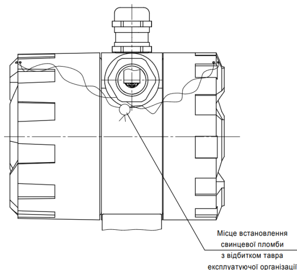
Рисунок 15 – Схема пломбування термінала багатофункціонального Vega-TM-2, термінала багатофункціонального Vega-TM-3, термінала багатофункціонального Vega-TM-4, термінала багатофункціонального Vega-TM-5, термінала багатофункціонального Vega-TM-6.
