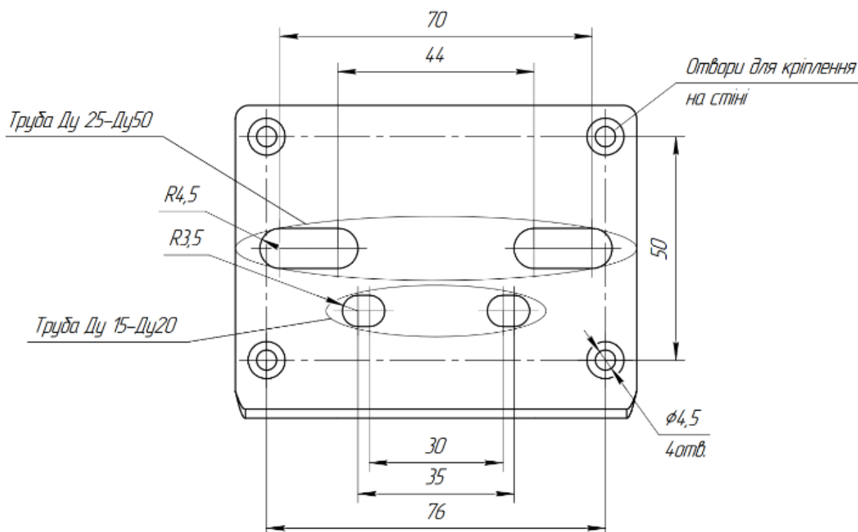
Рисунок 9 – Кронштейн для кріплення термінала Vega-TM-7
