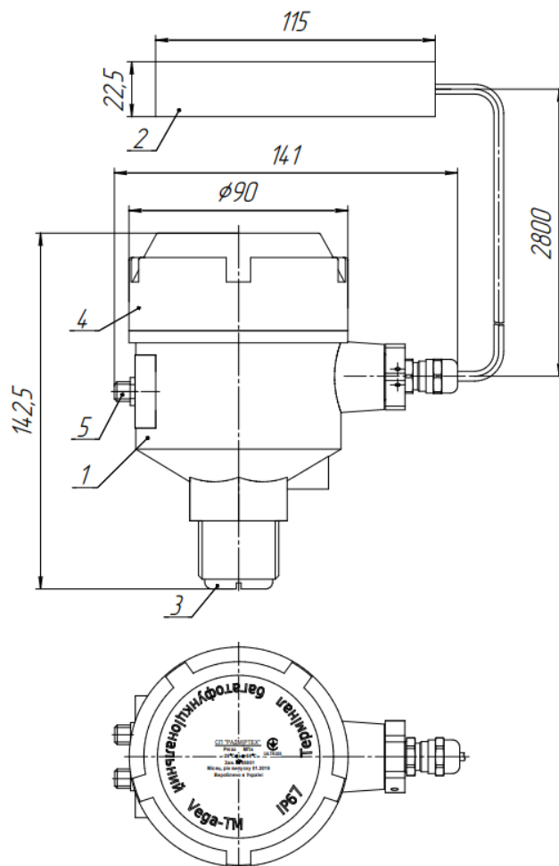
Рисунок 6 – Зовнішній вигляд та габаритні розміри термінала багатфункціонального Vega-TM-7
