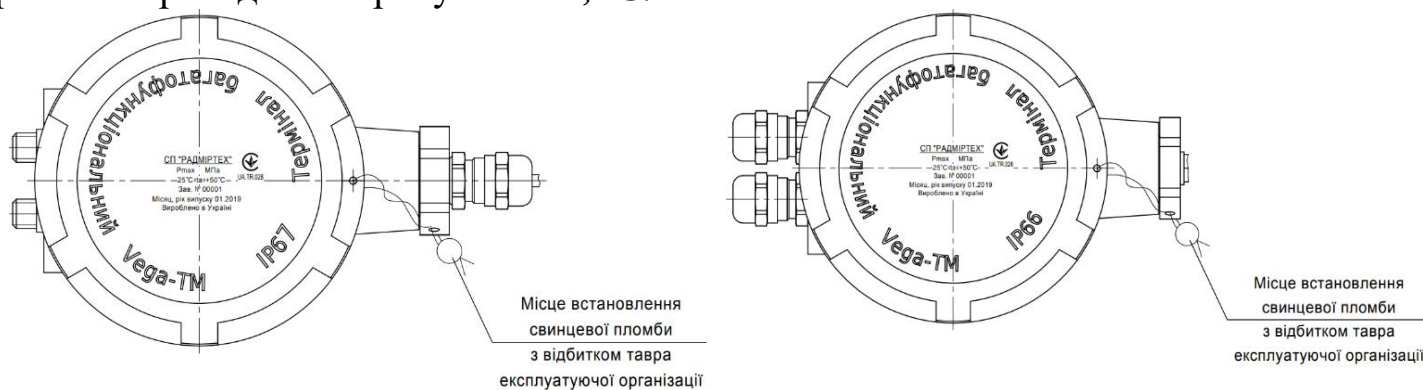
Рисунок 14 – Схема пломбування термінала багатофункціонального Vega-TM-0, термінала багатофункціонального Vega-TM-1 та термінала багатофункціонального Vega-TM-7
