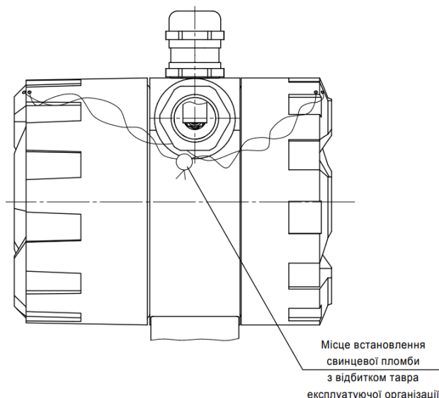
Рисунок 15 – Схема пломбування термінала багатофункціонального Vega-TM-2, термінала багатофункціонального Vega-TM-3, термінала багатофункціонального Vega-TM-5.
