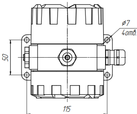
Рисунок 5 – Зовнішній вигляд та габаритні розміри термінала багатофункціонального Vega-TM-3, термінала багатофункціонального Vega-TM-5
