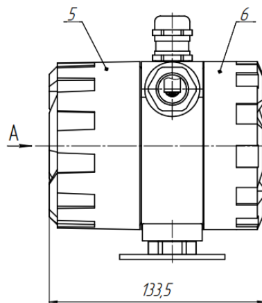
Рисунок 4 – Зовнішній вигляд та габаритні розміри термінала багатофункціонального Vega-TM-2
