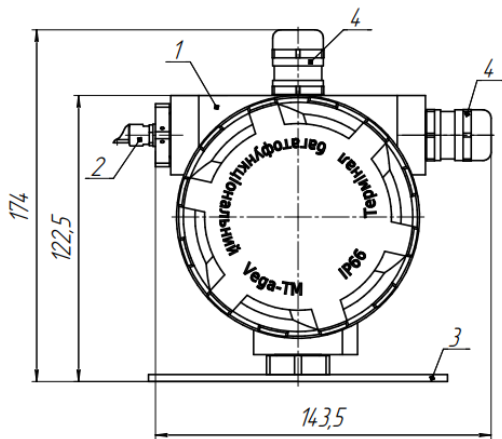
Рисунок 4 – Зовнішній вигляд та габаритні розміри термінала багатофункціонального Vega-TM-2
